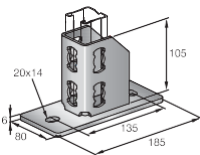
Base MQP-21-72 Itemn.: 369651
